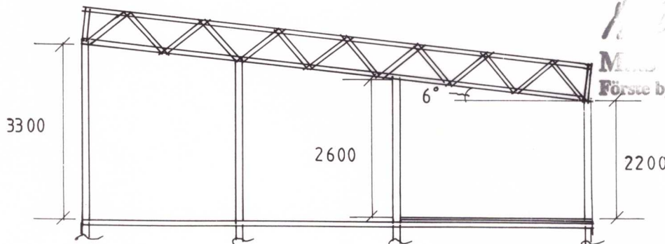
SEKTION A-A
